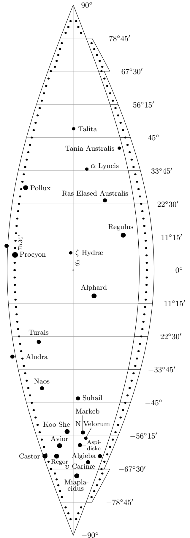
4 RA 7h 30' 9h 10h 30' 112.5° 135° 157.5°
