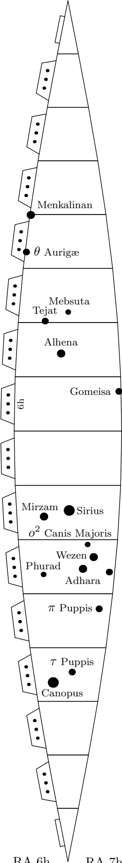
RA 6h RA 7h 30'
