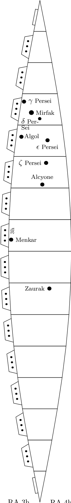
RA 3h RA 4h 30'
