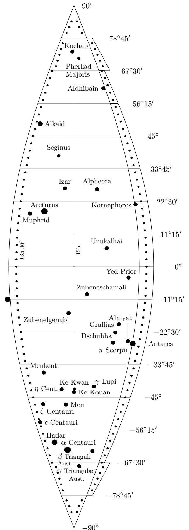
6 RA 13h 30' 15h 16h 30' 202.5° 225° 247.5°
