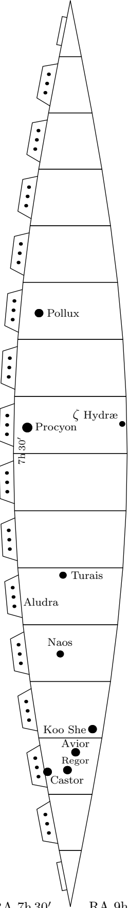
RA 7h 30' RA 9h
