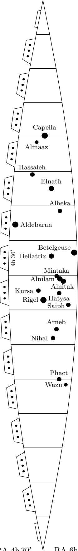
RA 4h 30' RA 6h
