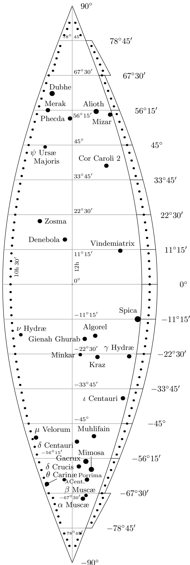
5 RA 10h 30' 12h 13h 30' 157.5° 180° 202.5°
